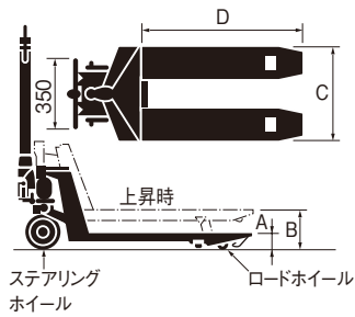
寸法図
