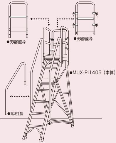
※イラストはMUX-PI1405（階段両手摺天場三方付き）です。
